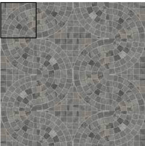
СХЕМА УКЛАДКИ 2
